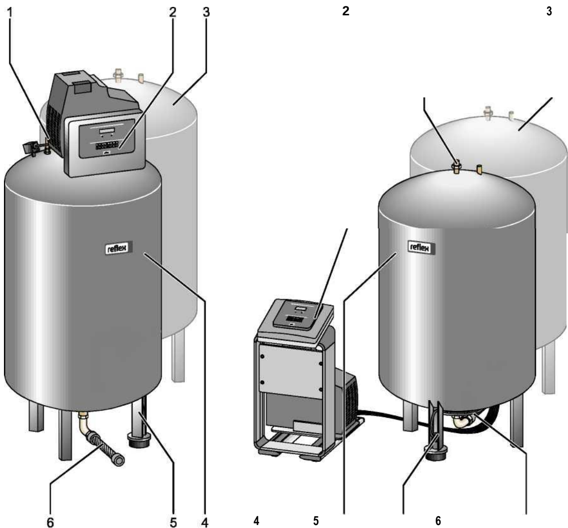
Reflexomat RS 90 /1 в компактном исполнении
