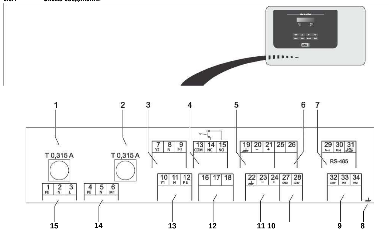
6.5.1 Схема соединений
